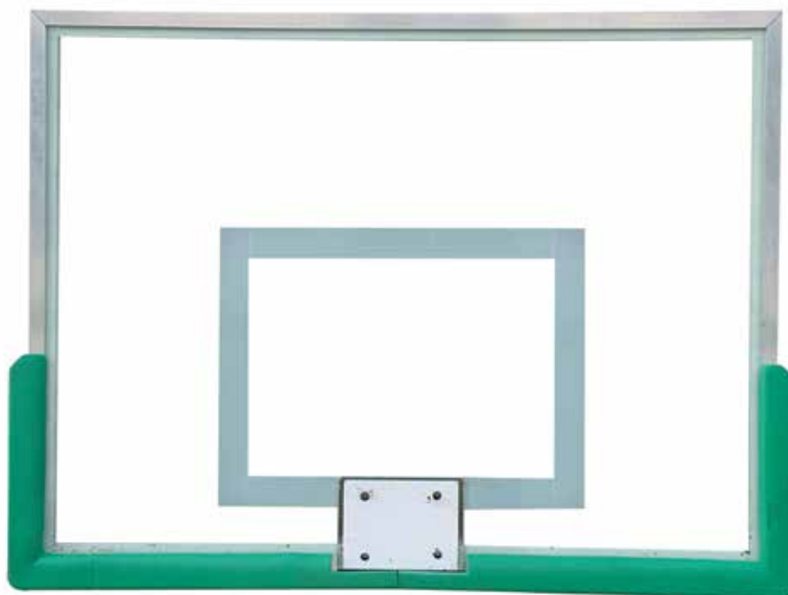
680 601 Tablero basket de cristal templado de 180 x 105 x 1,2 cm con protecciones. Tempered glass basket backboard with protections. 180 x 105 x 1,2 cm.
