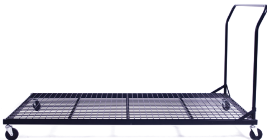
900895 Carro Porta-Colchonetas 2000 x 1000 mm. NUEVO MODELO Fabricado con acero tratado para la corrosión. 4 ruedas de PU, 2 fijas y 2 giratorias. Medidas de 2000 mm x 1000 mm. Plegable. Peso máximo recomendado 250 Kg. Trolley for Mats 2000 x 1000 mm. NEW MODEL. Made of steel treated for corrosion. 4 PU wheels (2 fixed and 2 swivel). Measures 2000 mm x 1000 mm. Foldable. Maximum weight: 250kg
